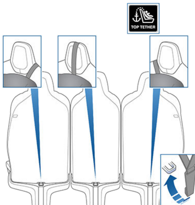
Correa sencilla - Segunda fila de asientos de banco
